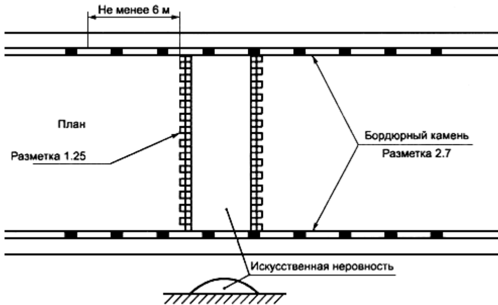
Рисунок 4 - Пример нанесения разметки 1.25 и 2.7 при устройстве ИН
